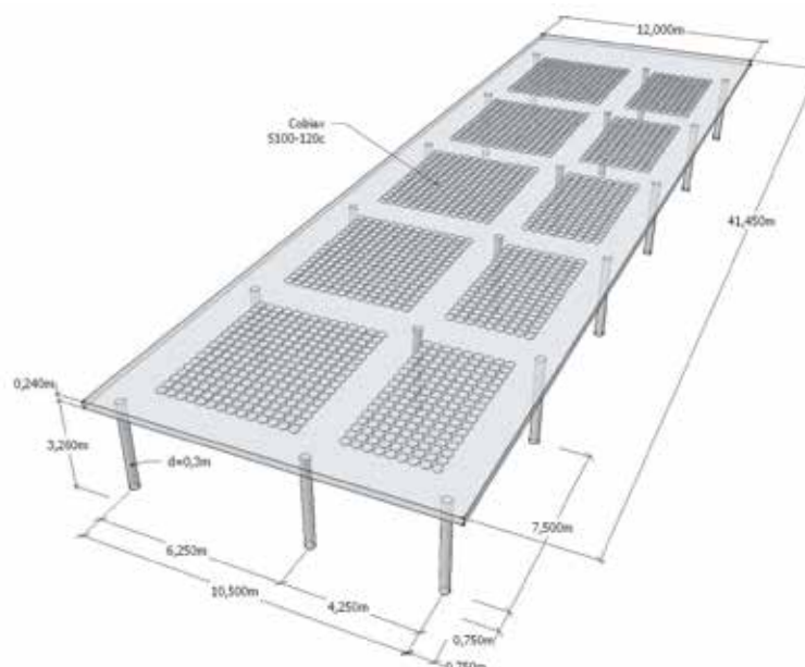
1b: Variante A319 - Cobiax-Decke, 24 cm Flachdecke (Spannweiten: 6,25 m / 4,25 m)
