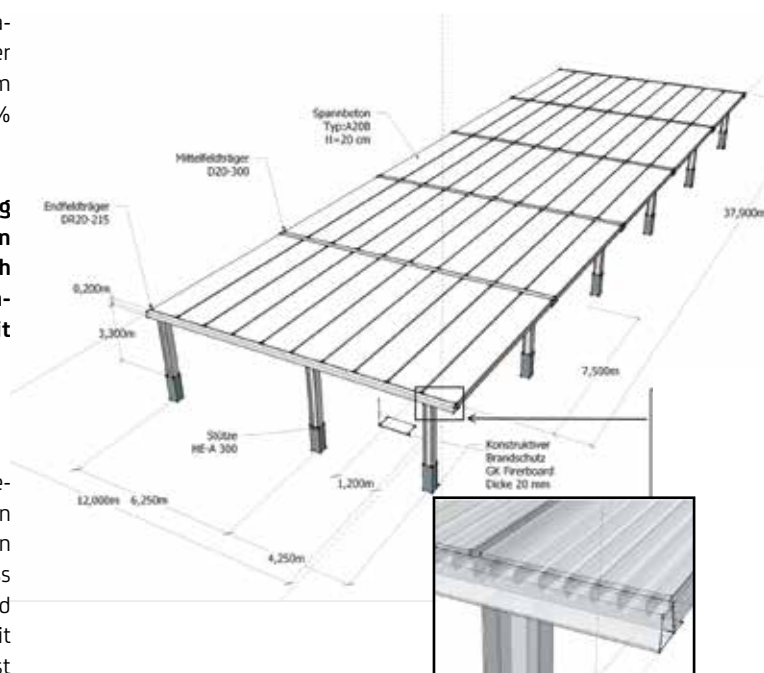
1c: Variante A315 BRESPA®-Decke A20B, 20 cm Flachdecke, Spannrichtung längs (Spannweiten: 7,50 m)
