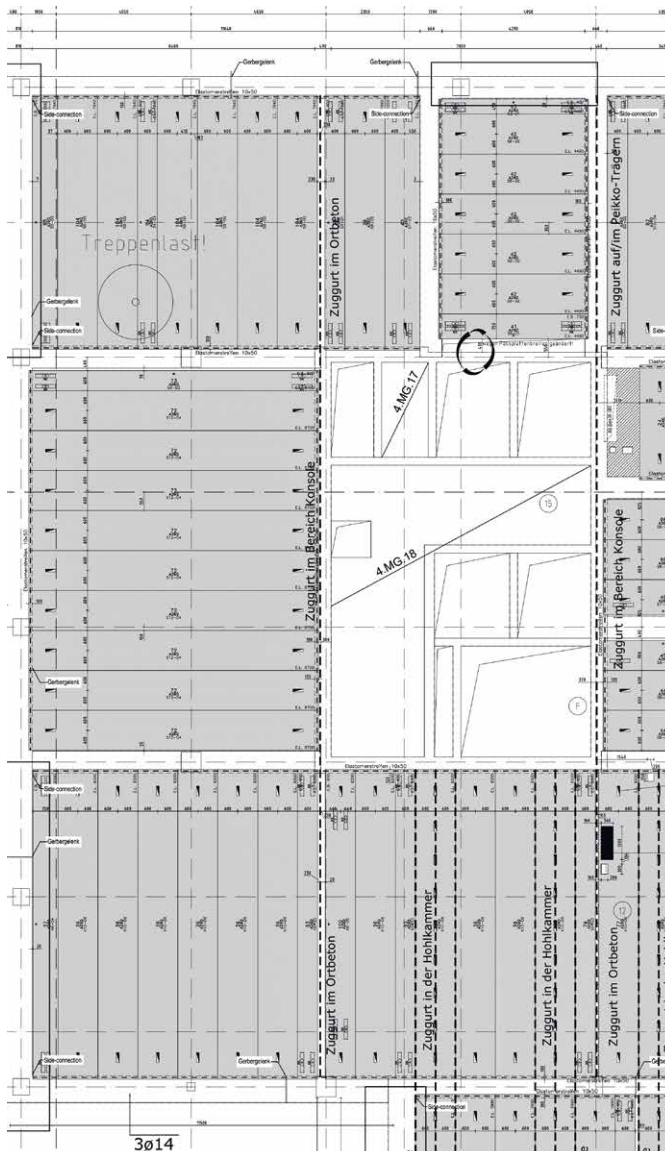
Bild 7 Ausschnitt aus dem EG-Deckenverlegeplan für den Gebädeturm
