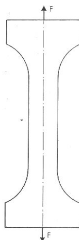
Bild 2: Belastungsanordnung Zugversuch
