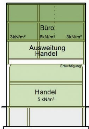
Abbildung 4.14 Zonenübergreifende Ausweitung von Nutzflächen und Auswirkungen auf die Konstruktion
