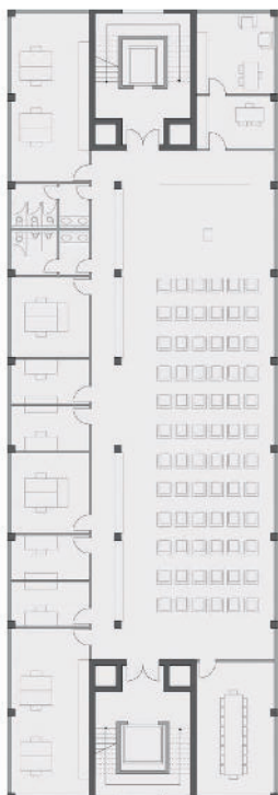
Abbildung 4.5 Nutzungsvarianten Regelgeschoss (Zone I)
