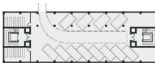
Bild 3 - Untergeschoss, Nutzungsszenario Tiefgarage
